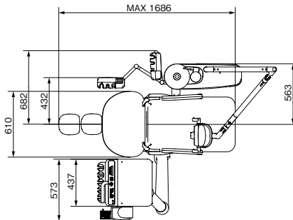
平面図 寸法(1/50縮寸)単位:mm
